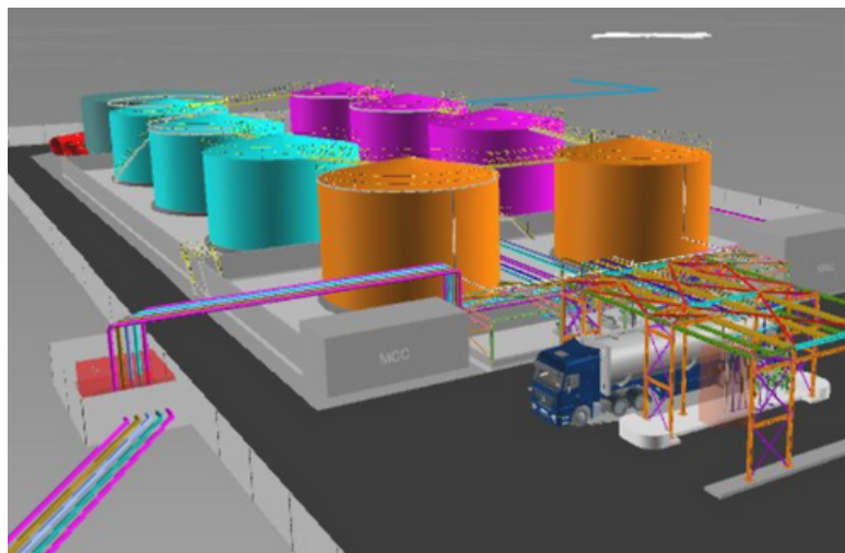
Een basis design van de nieuwe terminal met 8 tanks van ong. 1000 m 3
